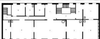
Store Kongensgade 68, 1. Sal. Planlægning udarbejdet efter tegninger i Københavns Kommunes Byggesagsarkiv og Brandtkaafens i Ripsarkivet
